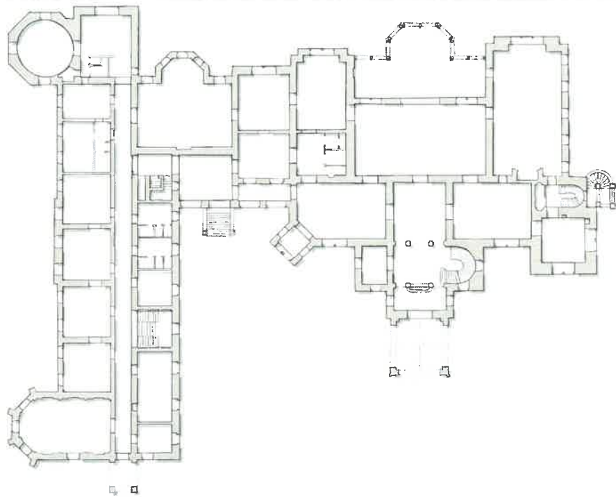
A kastély földszinti alaprajza a helyreállított télikerttel.
